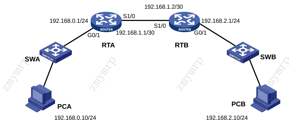
图2-1 实验组网图
